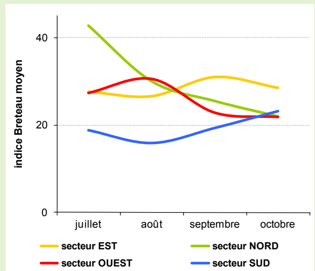
Figure 2 : Indice de Breteau moyen par mois et par secteur entre juillet et octobre 2012 à La Réunion
